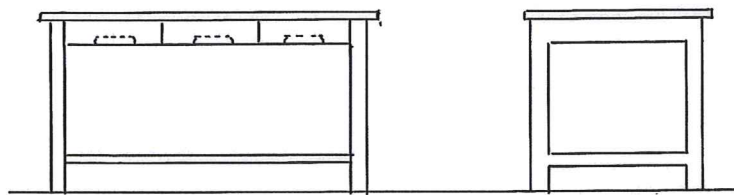
..... ㉡ 型作業台 (抽斗付)
