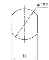
切欠図
