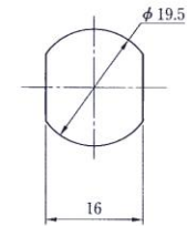
切欠図
