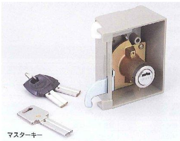
写真：MFLK1型
